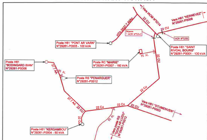
SCHEMA HTA AVANT TRAVAUX
